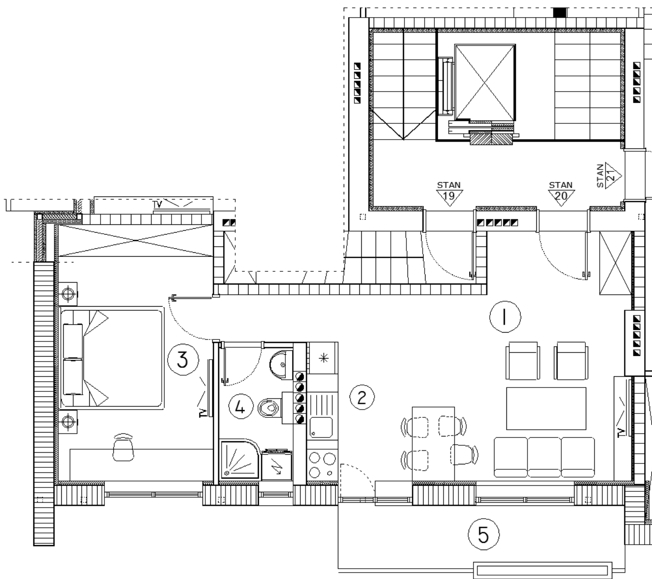
Osnova stana #20 sa oznakama prostorija
